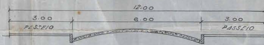
SEÇÃO DAS RUAS ESC. 1:100
