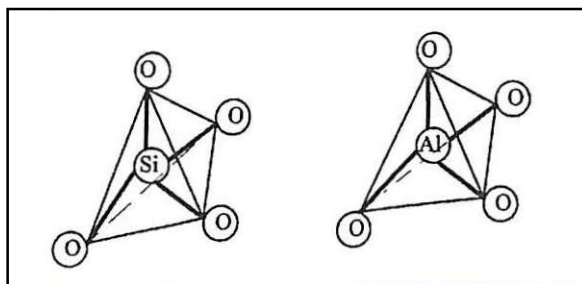
Figura 2 - Tetraedros de silício e alumínio (BRECK, 1974)
