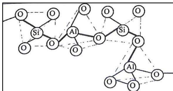
Figura 3 - Arranjo Estrutural dos tetraedros (BRECK, 1974)
