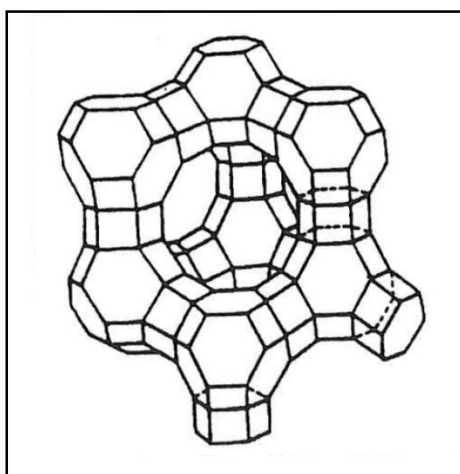
Figura 10 - Estrutura da zeólita Y (BRECK, 1974).
