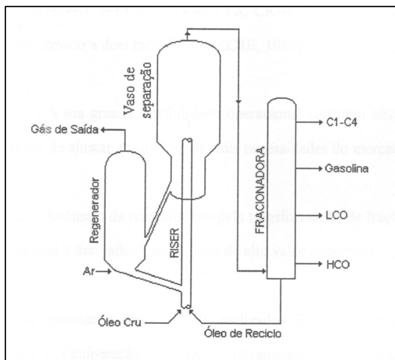
Figura 1 - Esquema simplificado do Processo de FCC (ABADIE, 1985).
