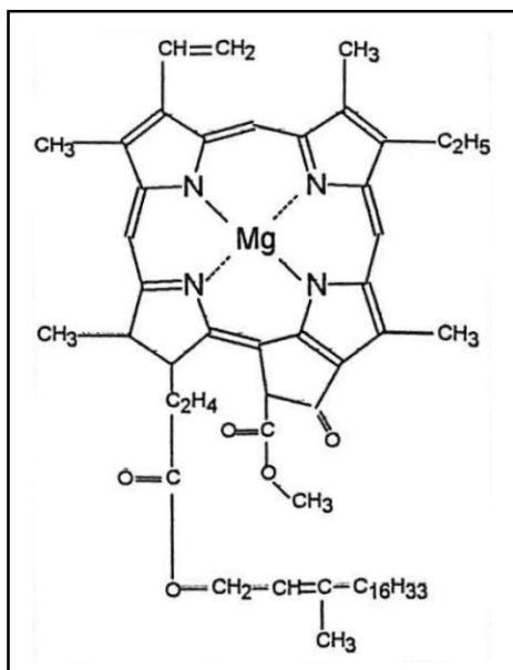
Figura 11 – Estrutura da Clorofila
