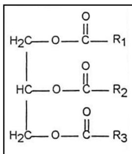
Fig. 12 – Molécula de triglicerídeo
