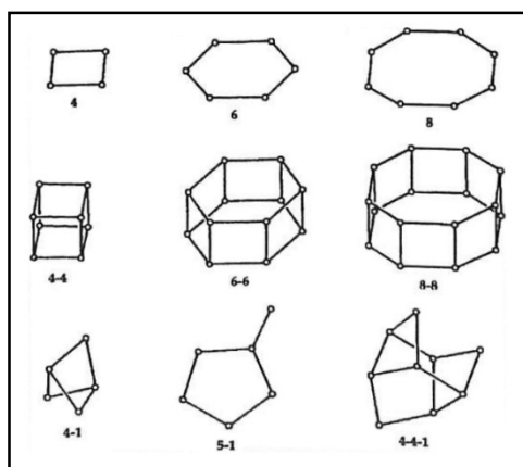
Figura 4 - Unidades Secundárias de Construção (GIANNETO, 1990).
