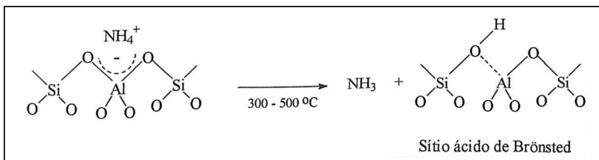
Equação 1 - Formação de sítios ácidos de Brønsted por decomposição térmica da forma amoniacal (GIANNETO, 1990).
