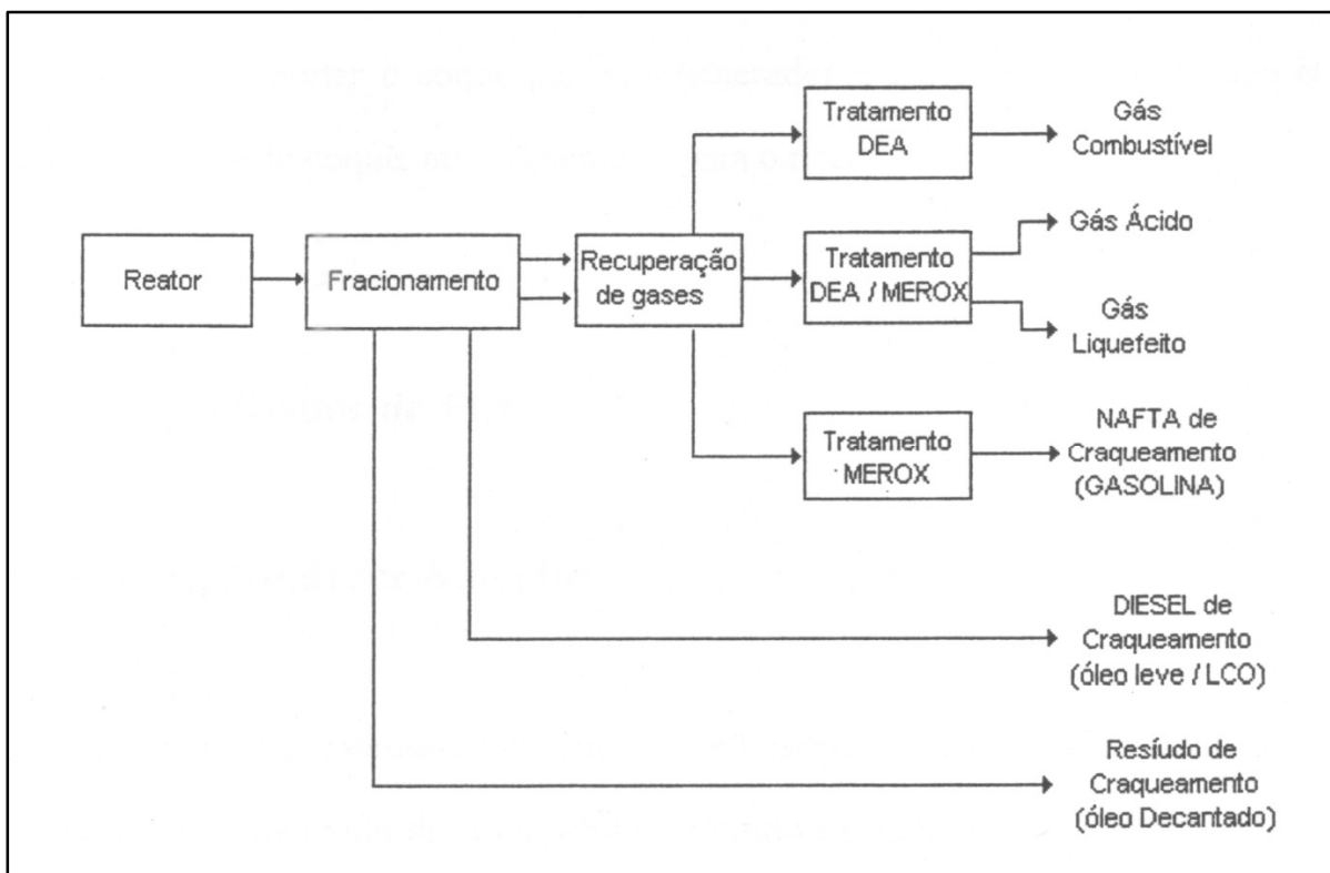
Esquema 1 – Processo de FCC, tratamento dos efluentes gasosos (ABADIE, 1985)
