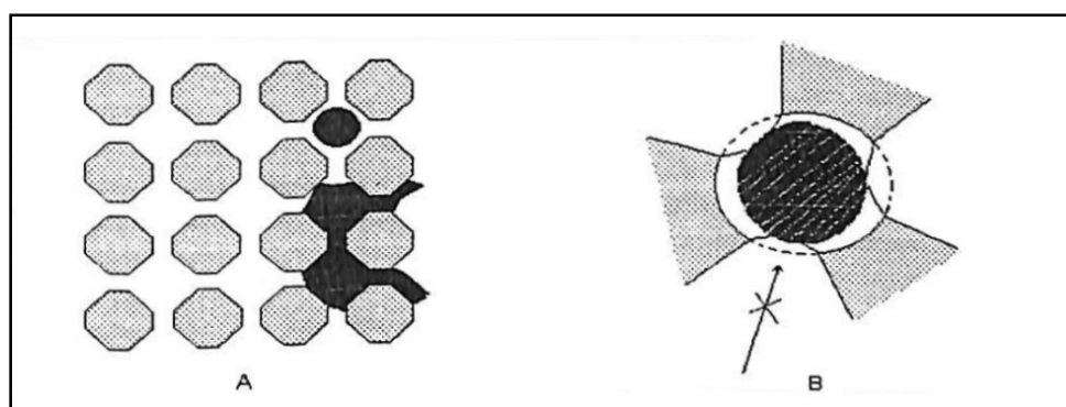
Figura 13 – (A) processo de obstrução dos poros pela formação de coque (B) Acesso à cavidade impedido devido à presença de coque.
