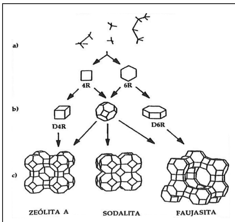
Figura 6 – Estruturas zeolíticas (BRECK, 1974)
