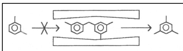
Figura 9 – Seletividade ao Estado de Transição (GIANNETO, 1990).
