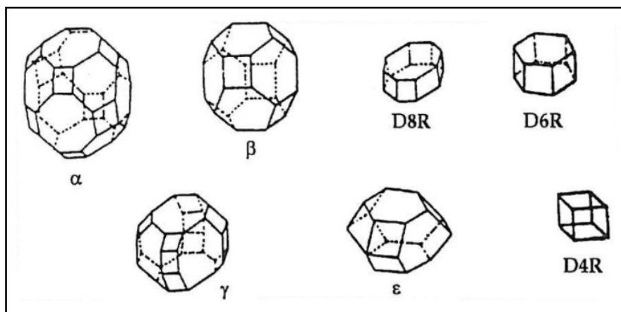
Figura 5 - Alguns poliedros presentes nas estruturas zeolíticas (GIANNETO, 1990): \alpha ou cubo octaedro truncado; \beta ou octaedro truncado; D8R ou anel duplo de 8 membros; D6R ou anel duplo de 6 membros (prisma hexagonal); \gamma (18-edro); \epsilon (11-edro); D4R ou anel duplo de 4 membros.
