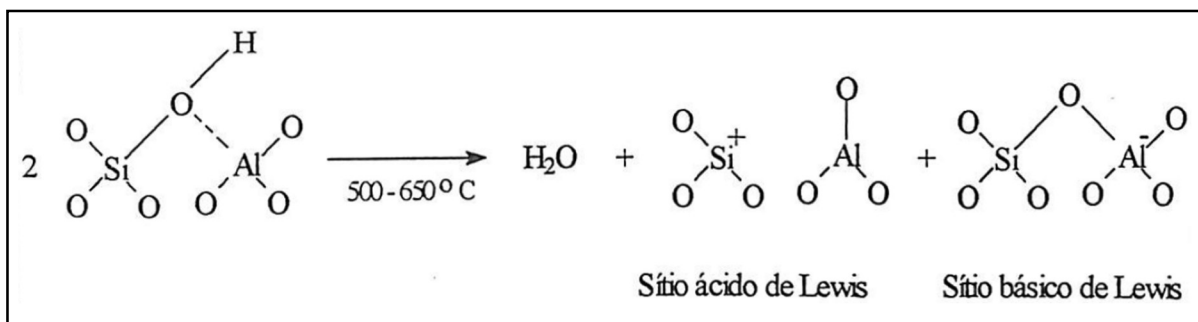
Equação 2 - Formação de Sítios de Lewis por desidratação térmica de zeólitas decationizadas (GIANNETO, 1990).
