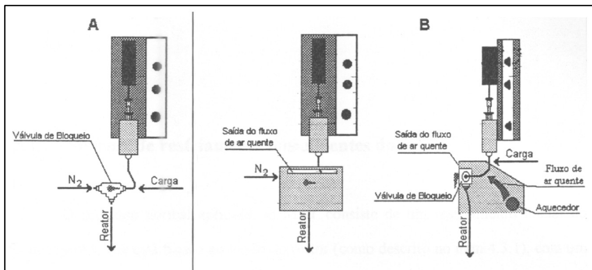
Figura 16 – (A) Sistema de injeção sem proteção e aquecimento, (B) visão frontal e lateral de sistema de injeção com proteção e aquecimento
