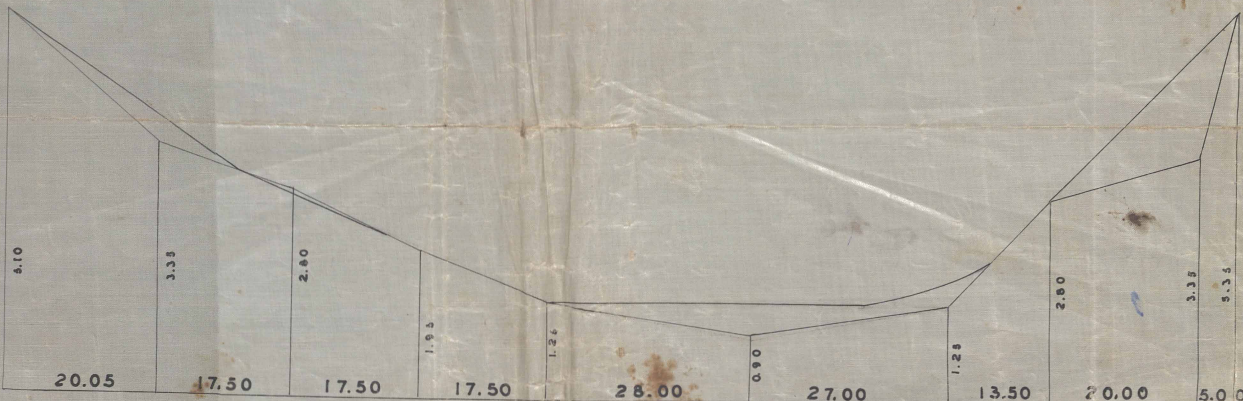
RUA CRUZEIRO DO SUL PERFIL LONG.
