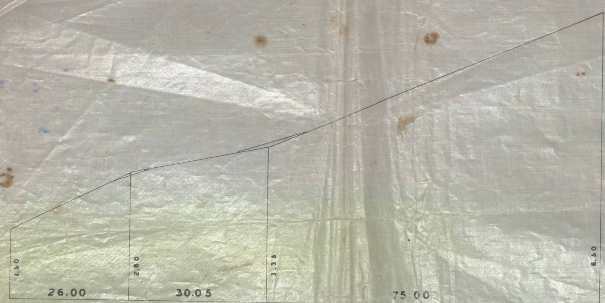
RUA N. S. DE FÁTIMA PERFIL LONG.
