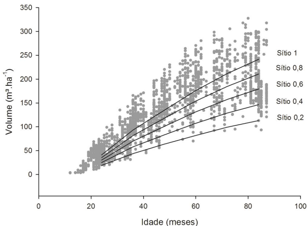
Figura 11. Curvas de produção em volume em relação a idade nas diferentes classes de sítio para região de Bocaiúva (MG) oriundas do modelo 3-PG.
